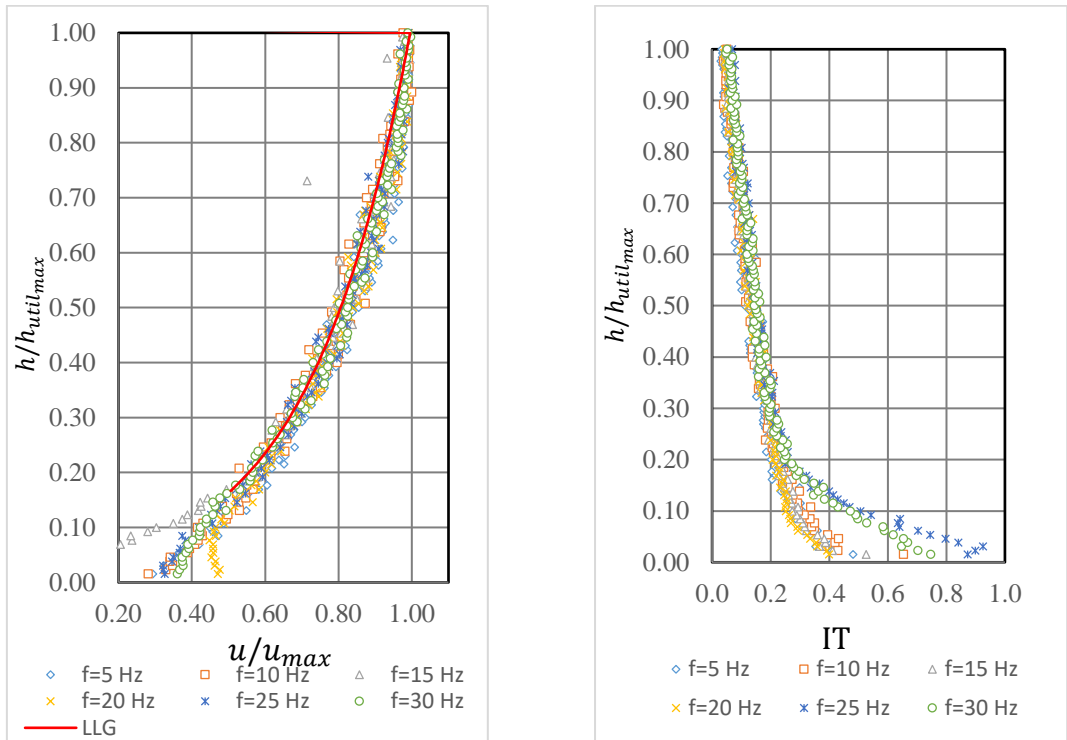
Distribuiii de viteze adimensionalizate funcie de viteza maximă (inclusiv curba teoretică) și intensitate turbulenta în vena de măsură, pentru dimensiunea rugozitatilor RV=10\text{ cm} (masurate in aval TA Etapa I -2018)
